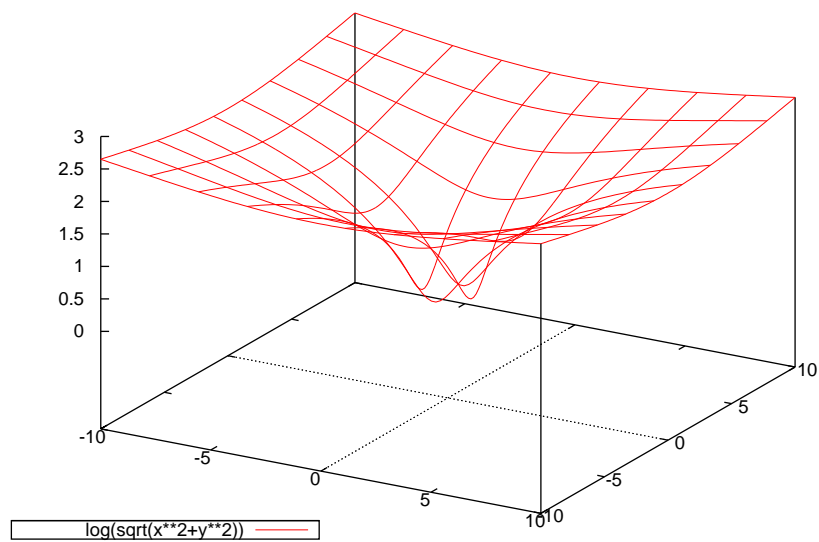
Figura 7: Gráfico 3d
