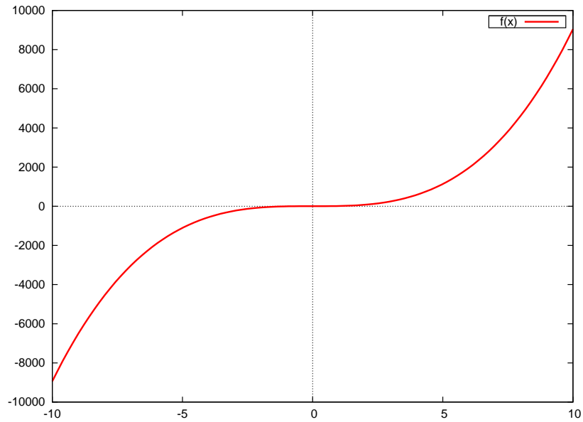
Figura 15: Função Polinomial
